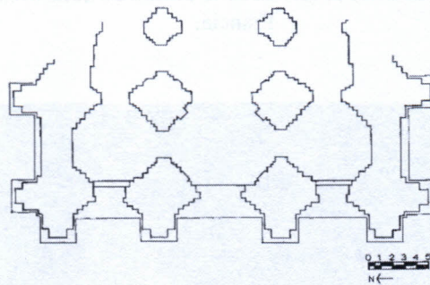
Ilustración 42. Planta del cuerpo occidental de la iglesia de Saint Denis, Francia (dibujo de (Crosby, 1968, 41)).
