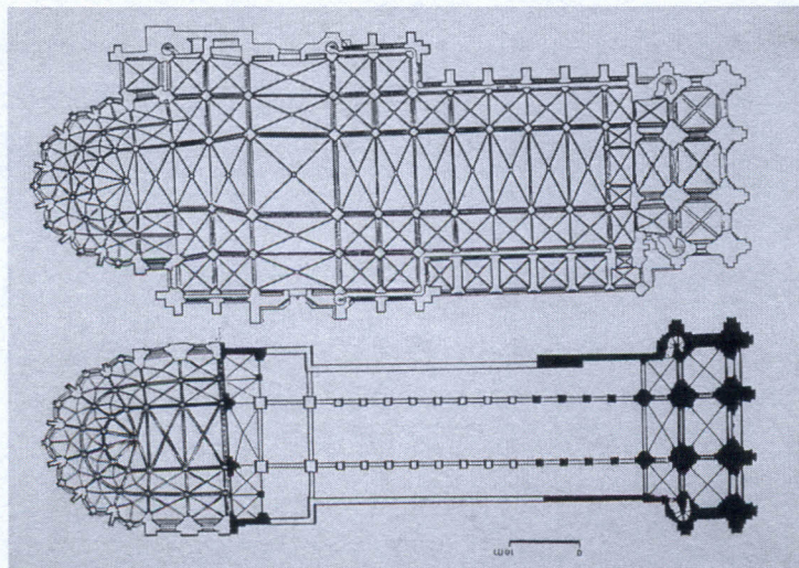
Ilustración 32. Planta de la Abadía de Saint Denis. Arriba: estado actual. Abajo: siglo XII, durante la época del abad Suger.
