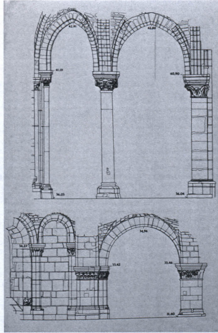
Ilustración 85. Elevación de la cripta y del chevet de la iglesia de Saint Denis, capilla radial.
