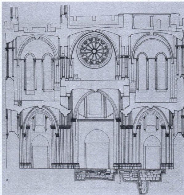
Ilustración 49. Sección transversal de las bahías internas del nártex y de la fachada occidental de la iglesia de Saint Denis, ca. 1135-1140. Francia.
