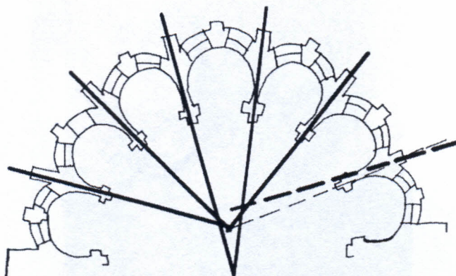
Ilustración 89. Planta de la cripta de la iglesia de Saint Denis que muestra la inclinación de los contrafuertes.
