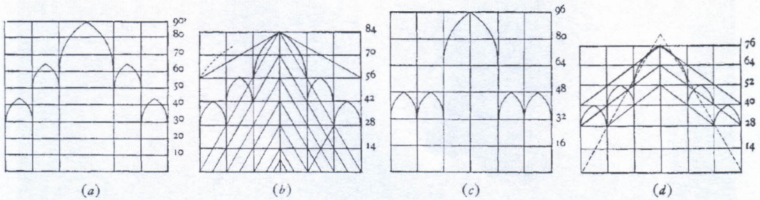
Ilustración 17. Catedral de Milán. Proyectos para determinar las proporciones y la altura de la nave, los pasillos, pilares y bóvedas, a construir sobre cimientos de 90 braccie de ancho. (a) Proyecto de 1390 empleando unidades de 10 braccie , según bosquejo y notas de Antonio di Vicenzo. (b) Proyecto de 1391 empleando unidades de 14 braccie , inscrito dentro de un marco establecido por triángulos equiláteros, según boceto de Gabriele Stornaloco. (c) Proyecto de 1392 a partir de una rejilla de cuadrados, reconstruido según evidencia textual por James Ackerman. Propuesto probablemente por Heinrich Parler de Gmünd. (d) Proyecto aceptado en 1392 empleando el proyecto de Stornaloco hasta una altura de 28 braccie (líneas punteadas), y continuado con unidades de 12 braccie inscritas dentro de un marco de triángulos pitagóricos, siguiendo las indicaciones del capítulo de la catedral.
