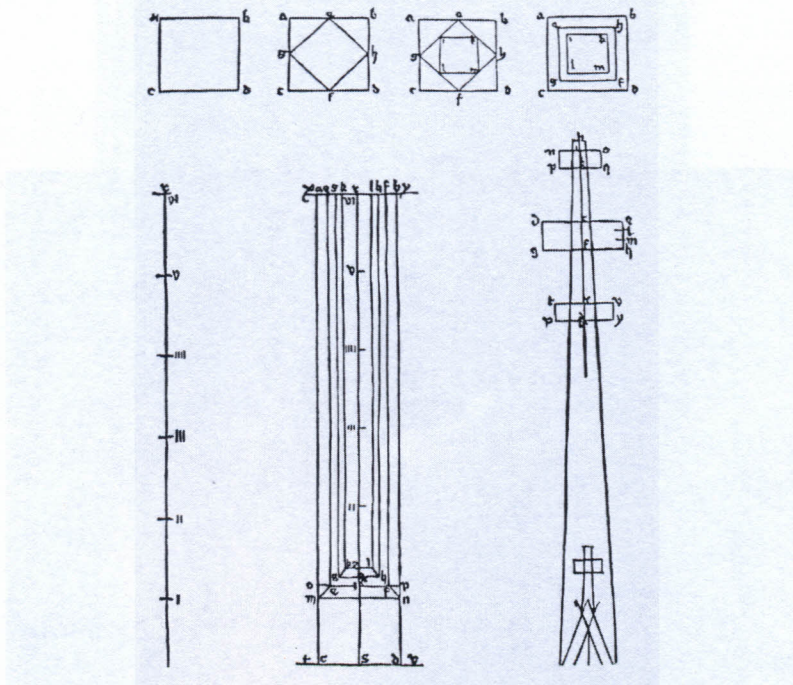
Ilustración 14. Pasos para dibujar un pináculo, según M. Roritzer.
