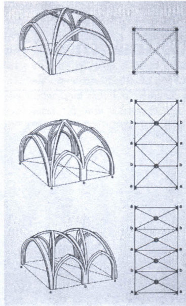
Ilustración 3. Tipos de bóvedas góticas.
