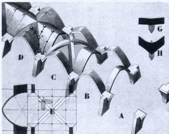
Ilustración 12. Elementos que constituyen una bóveda de crucería (A, B y C), esquema de funcionamiento y de transmisión de empujes (D y E) y secciones de los arcos diagonales de una bóveda de crucería (G y H) (Abraham, 1934b).
