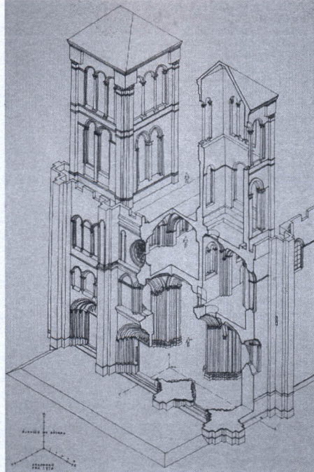
Ilustración 41. Reconstrucción isométrica de las bahías occidentales del nártex de la iglesia de Saint Denis, ca. 1135-1144. Francia.
